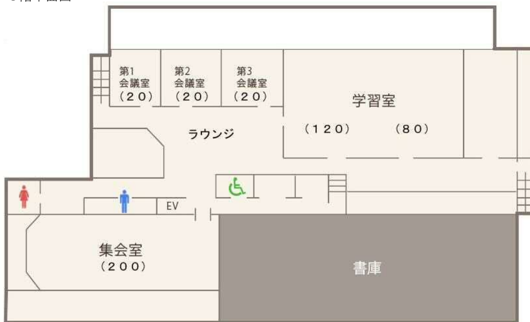
3階平面図
